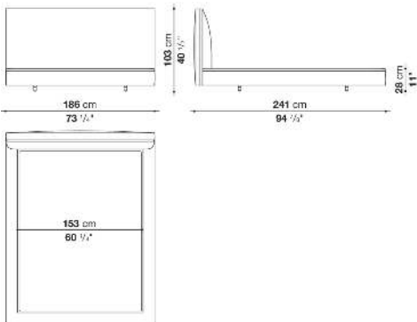
LRA153
